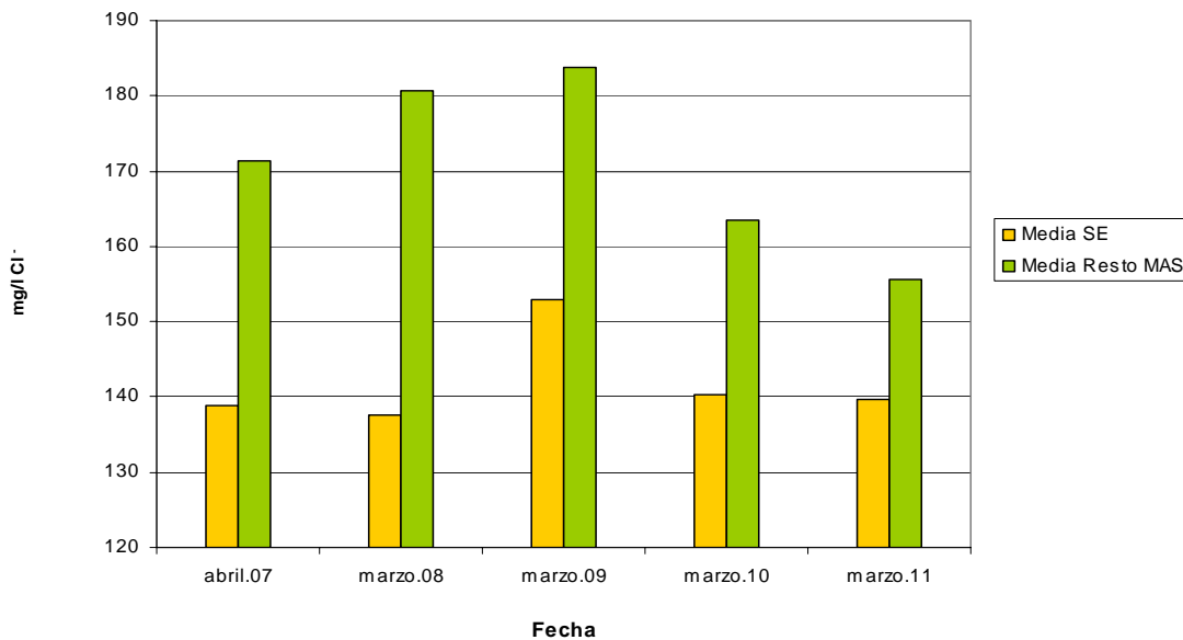
EVOLUCIÓN DEL CONTENIDO EN CLORUROS (VARIACIONES)- MAS 80.141 PLANA DE VALENCIA NORTE
