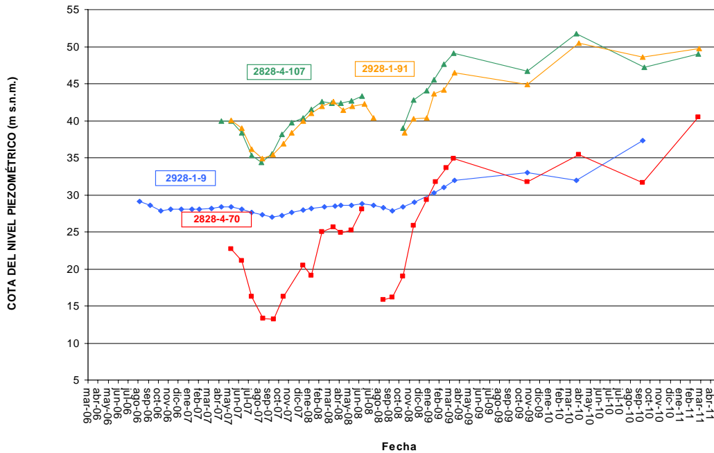
EVOLUCIÓN PIEZOMÉTRICA - MAS 80.141 PLANA DE VALENCIA NORTE Sector Torrente
