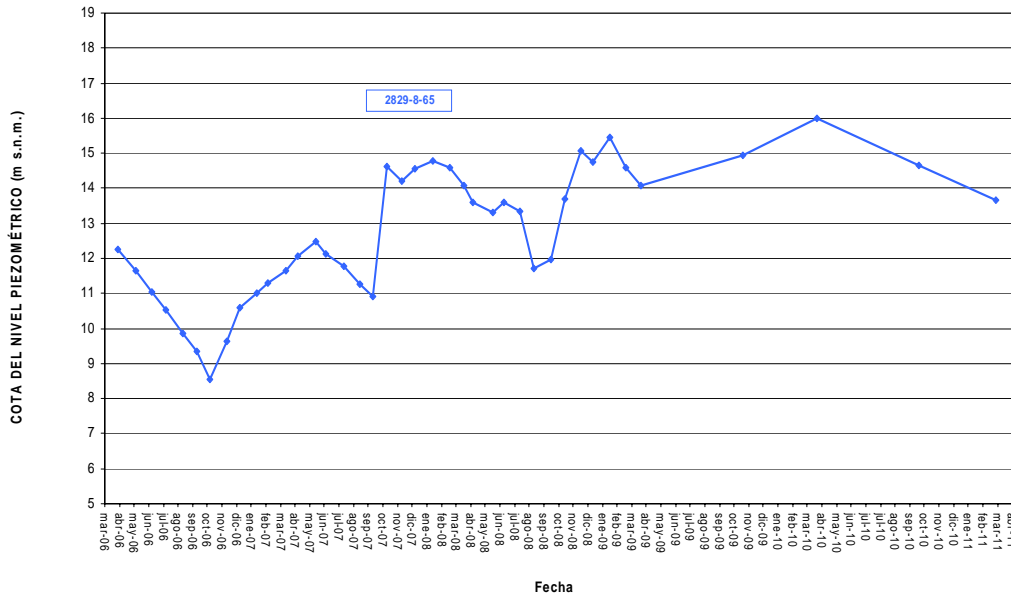
EVOLUCIÓN PIEZOMÉTRICA - MAS 80.142 PLANA DE VALENCIA SUR Sector Benimodo
