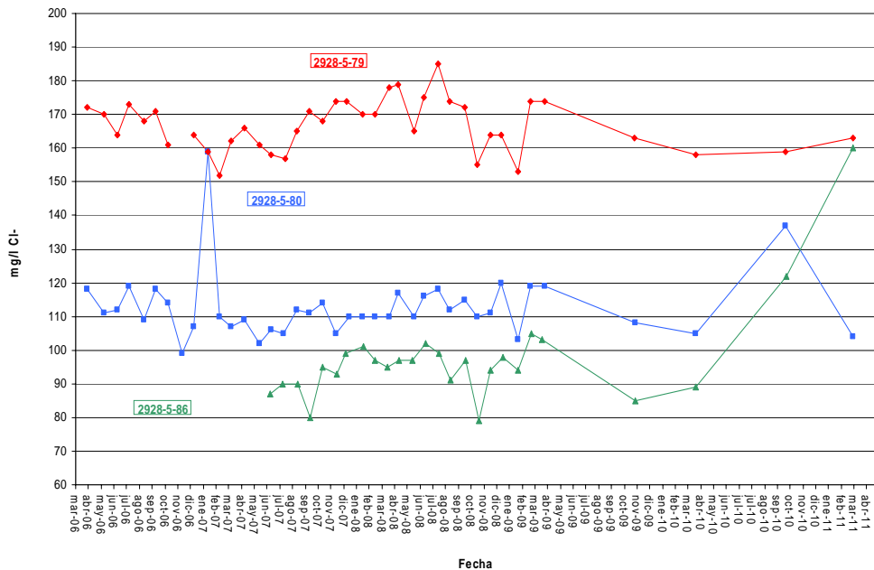
EVOLUCIÓN DEL CONTENIDO EN CLORUROS - MAS 80.140 BUÑOL-CHESTE Sector Picassent Norte
