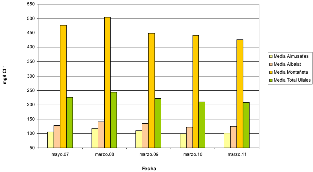
EVOLUCIÓN DEL CONTENIDO EN CLORUROS - ULLALES ALBUFERA
