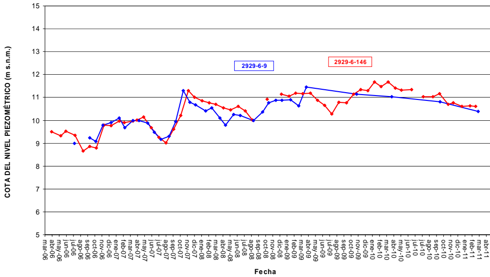
EVOLUCIÓN PIEZOMÉTRICA - MAS 80.142 PLANA DE VALENCIA SUR Sector Albalat
