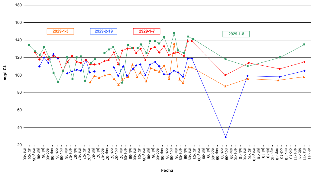
EVOLUCIÓN DEL CONTENIDO EN CLORUROS EN MAS 80.142 PLANA DE VALENCIA SUR Sector Albufera Sur
