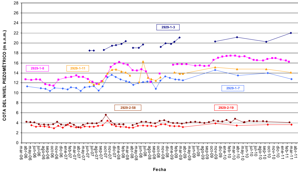
EVOLUCIÓN PIEZOMÉTRICA - MAS 80.142 PLANA DE VALENCIA SUR Sector Albufera Sur
